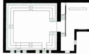
Grundriss
